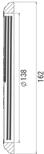
断面図 A-A
