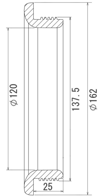
断面図 B-B
