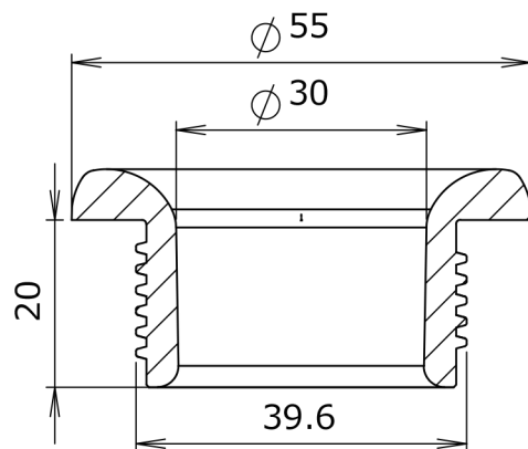
断面図 B-B
