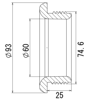
断面図 B-B
