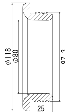
断面図 B-B
